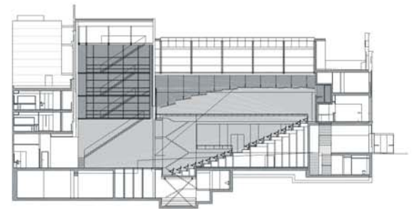
Secció teatre. E:1/700.
