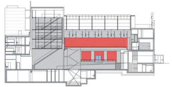
Secció ball. E:1/700.
