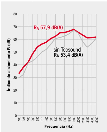
Gráfico comparativo de aislamiento acústico
