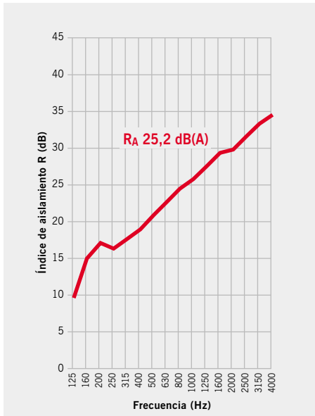
Gráfico de aislamiento acústico TECSOUND® 50
