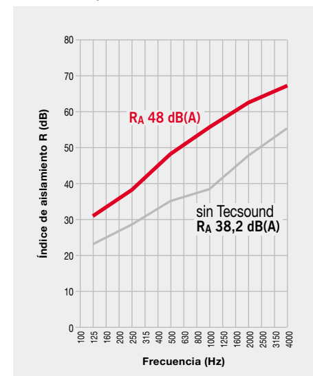
Gráfico comparativo de aislamiento acústico
