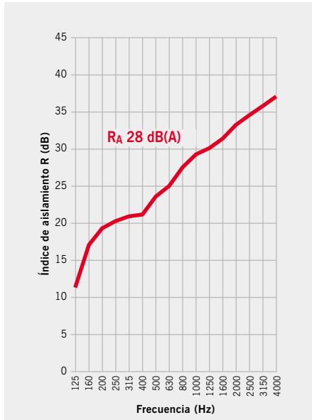
Gráfico de aislamiento acústico TECSOUND® 70
