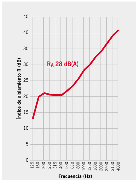
Gráfico de aislamiento acústico TECSOUND® FT 75
