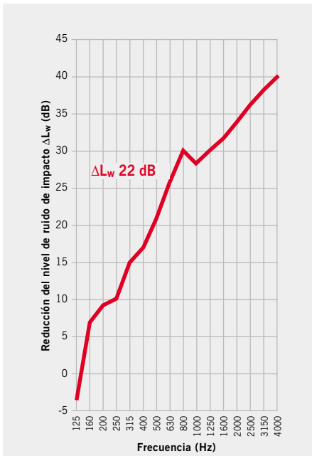
Gráfico de aislamiento a ruido de impacto TECSOUND® FT 75
