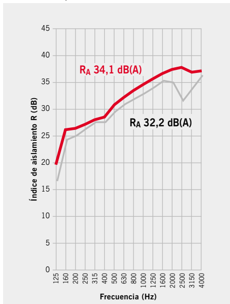
Gráfico comparativo de aislamiento acústico
