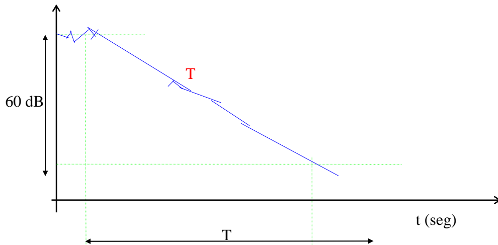
Figura 1.6: Forma de la curva de decaimiento tipo lineal campo difuso
