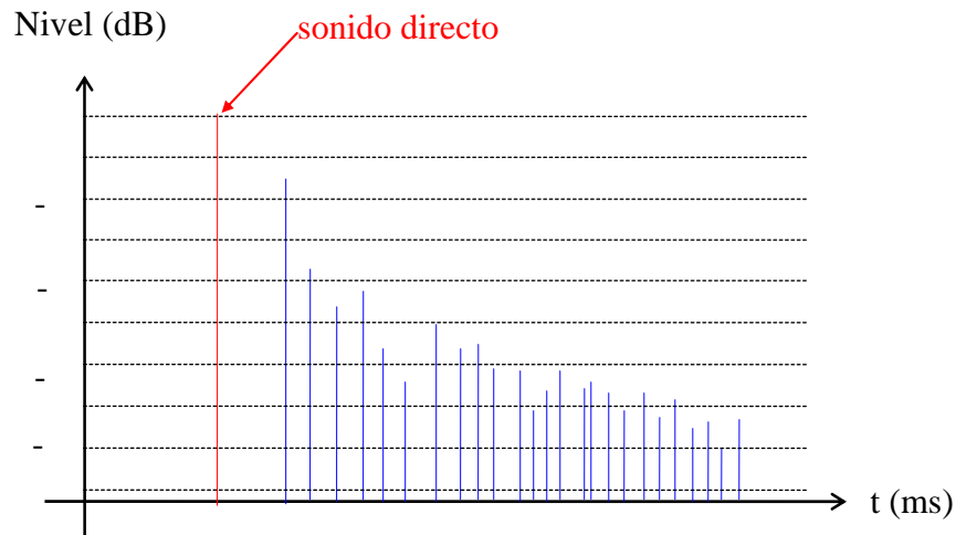
Figura 1.2: Ecograma de una sala
