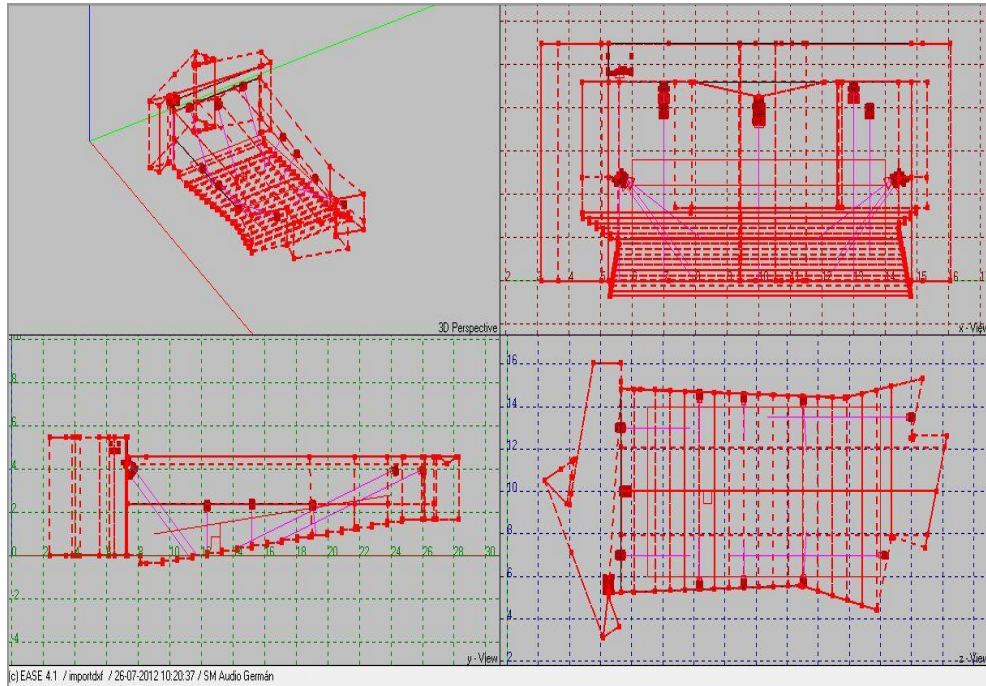
Figura 3.- Modelo arquitectónico para modelación de parámetros acústicos.
