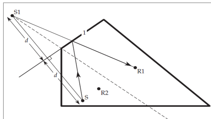
Figura 1.- Esquema referencial Fuente - Imagen "Mirror image".
