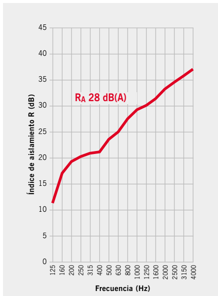
Gráfico de aislamiento acústico TECSOUND® 70
